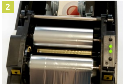
2 Foliendrucker anschließen und Metallic-Folie einlegen.
